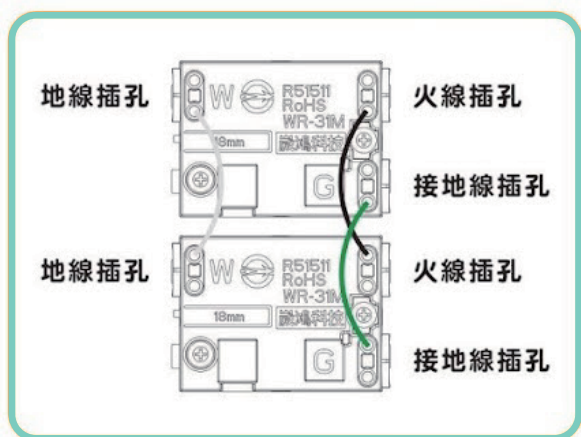
雙座配線圖
